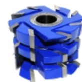
Фрезерные головки для задвижных ножей
